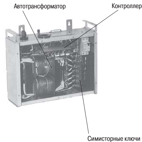
Рис. 8. Устройство стабилизатора
