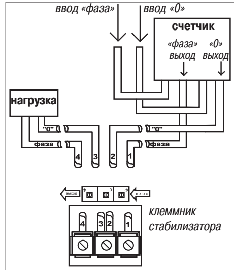
Рис. 17. Схема установки
